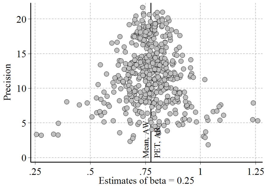
Figure 7. Case (2.1) the DGP = (2a), EM = (2b)
