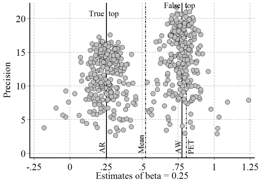
Figure 6. Case (1.1) the DGP = EM = (2a)
