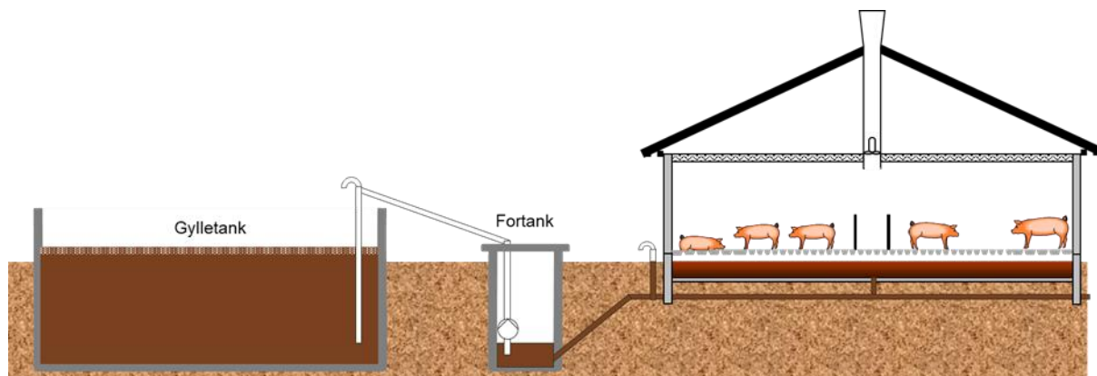
Figur 1. Principskitse af svinestald med tilhørende gyllesystem. Gyllen opsamles i gylle-kummen under spaltegulv i stalden. Fra stalden sluses gyllen ud til en fortank via et udslusningssted og et lukket rørsystem, og fra fortanken pumpes gyllen videre til gylletanken (Kilde: Peter Kai, Institut for Ingeniørvidenskab).
